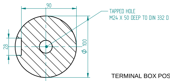
Przekrój A-A 1:2
